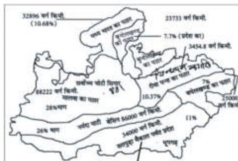
सतपुड़ा-मैकल पर्वतमाला
